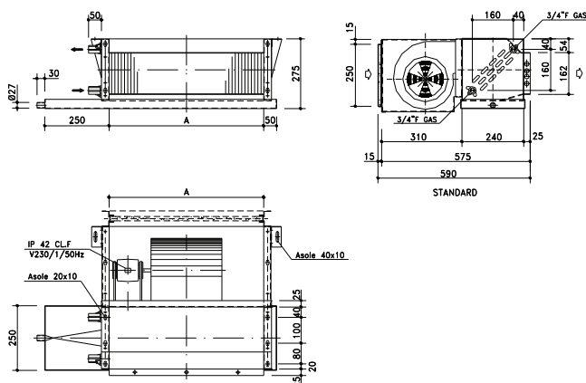
Габаритные размеры и масса
